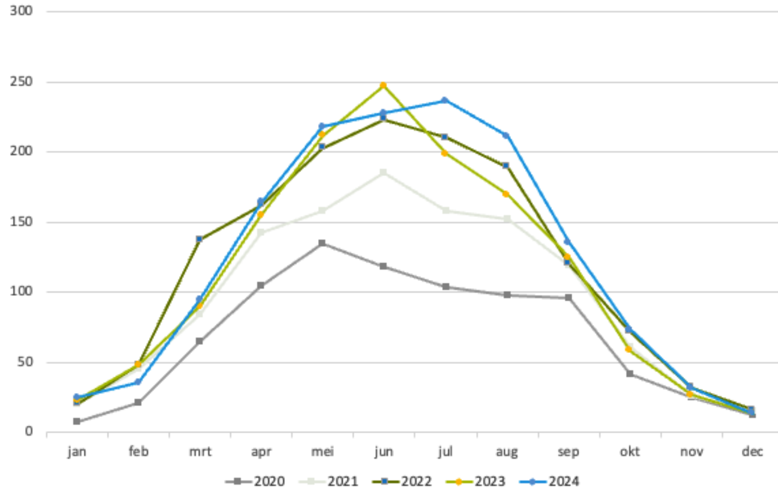
Opgewekte zonnestroom per maand 2024 (MWh)
